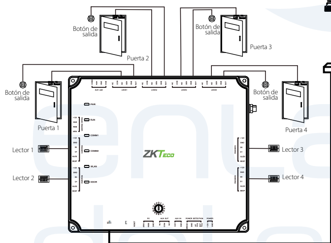
Control de entrada / salida de 4 puertas (Lectores Wiegand)
