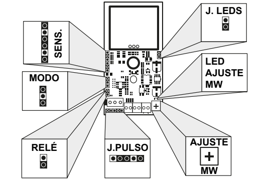
Identificación de los jumpers de ajustes
